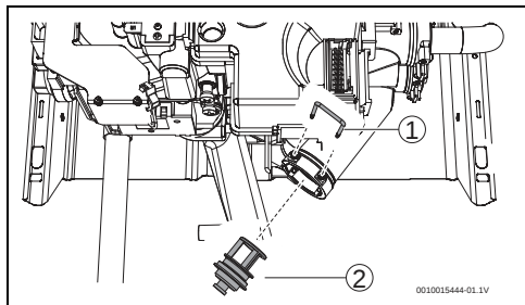
10. ábra Ürítés
