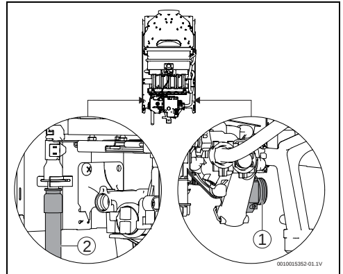
13. ábra Vízbekötés
